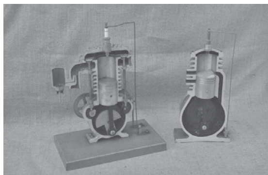
Εικόνα 4. Τομές βενζινοκινητήρα.
