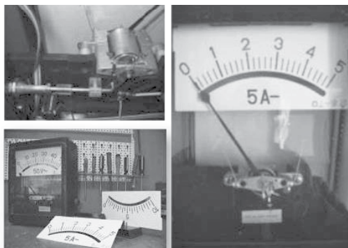
Εικόνα 3. Αναλογικό πολύμετρο μεταβλητής κλίμακας.
