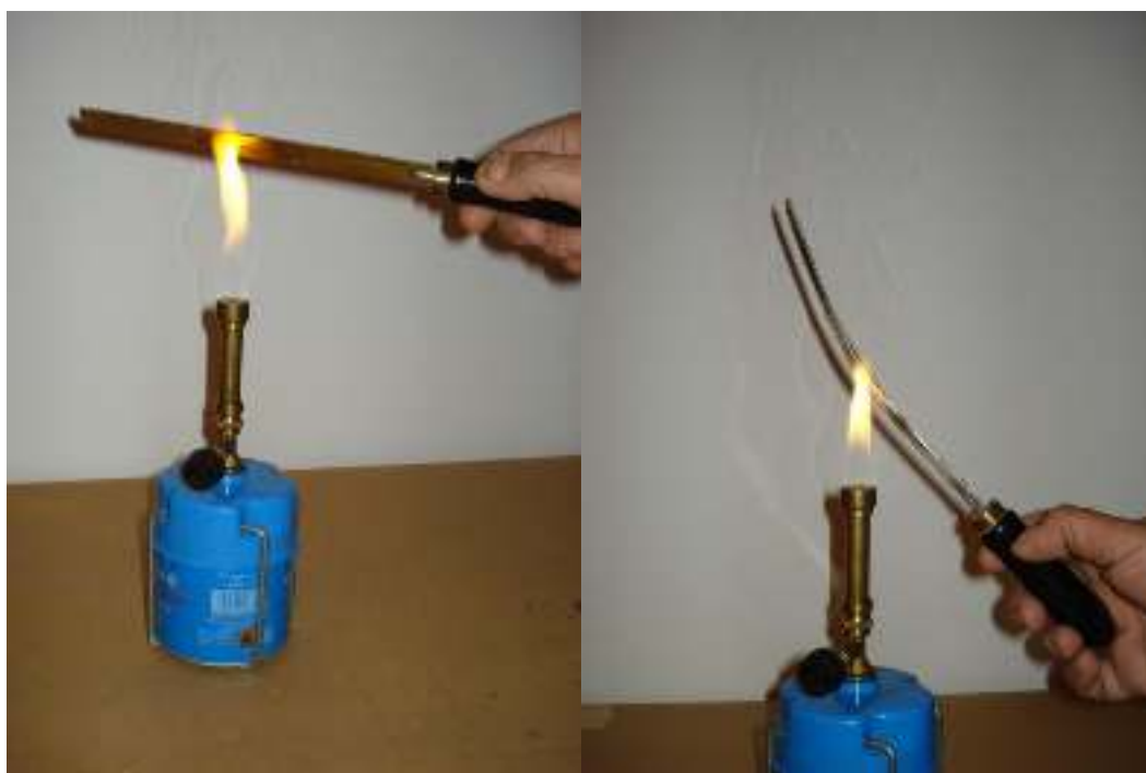
Διμεταλλικό έλασμα
